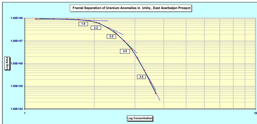
شکل ۳-۴: خطوط برازش شده به منحنی فرکتالی عیار-مساحت برای جدایش جوامع آنومالی و زمینه
